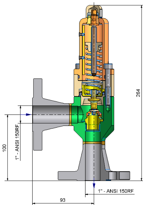
CF-R Flanschausführung CF-R flanged design
